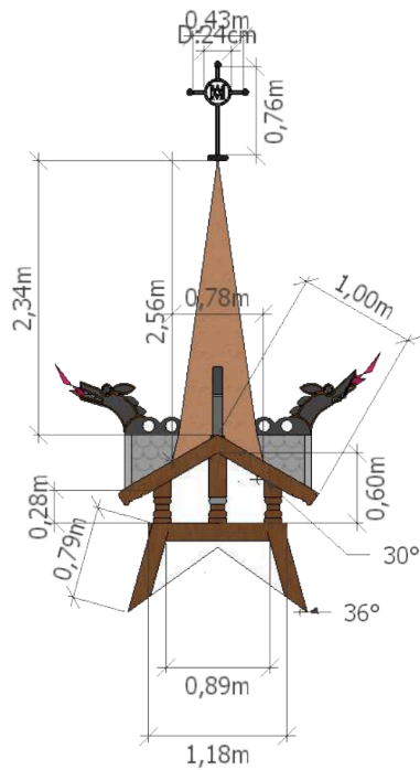
SNITT TÅRN
